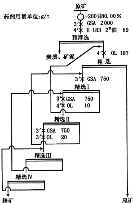
图 1 闭路试验工艺流程
