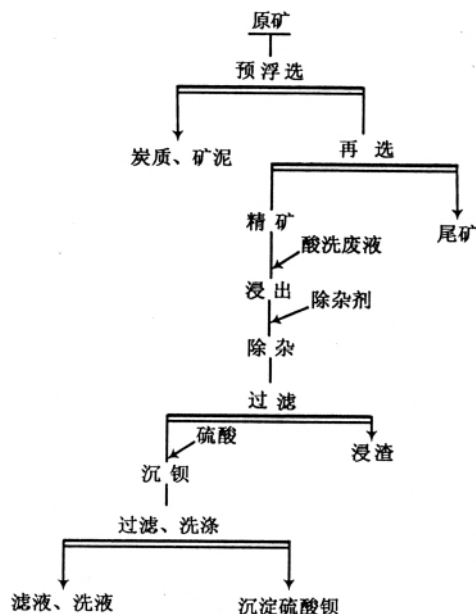
图2 制钡盐工艺流程图
